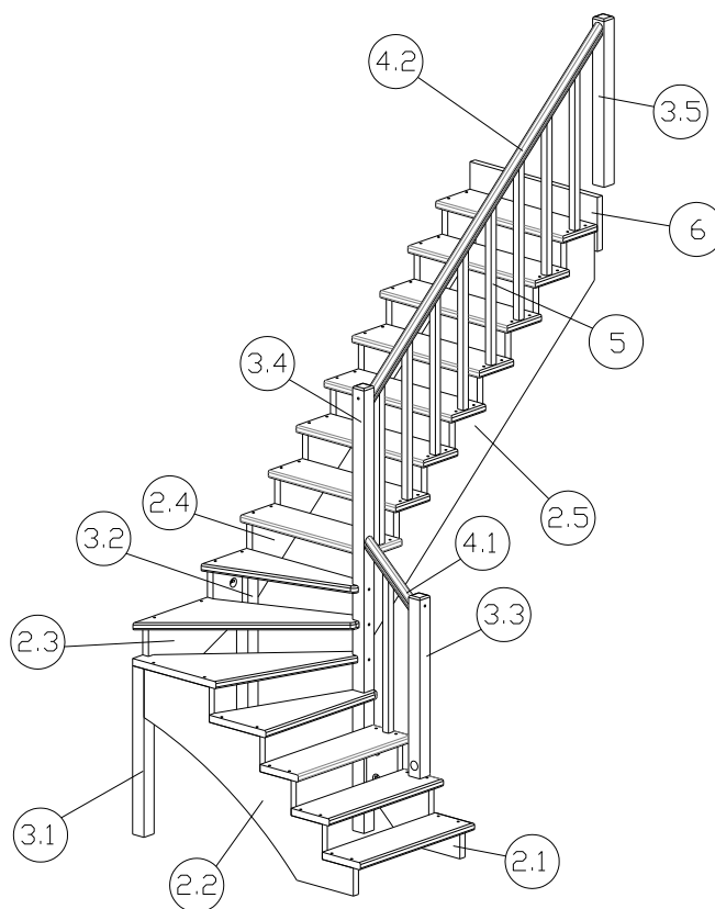
Вариант без подступеней
