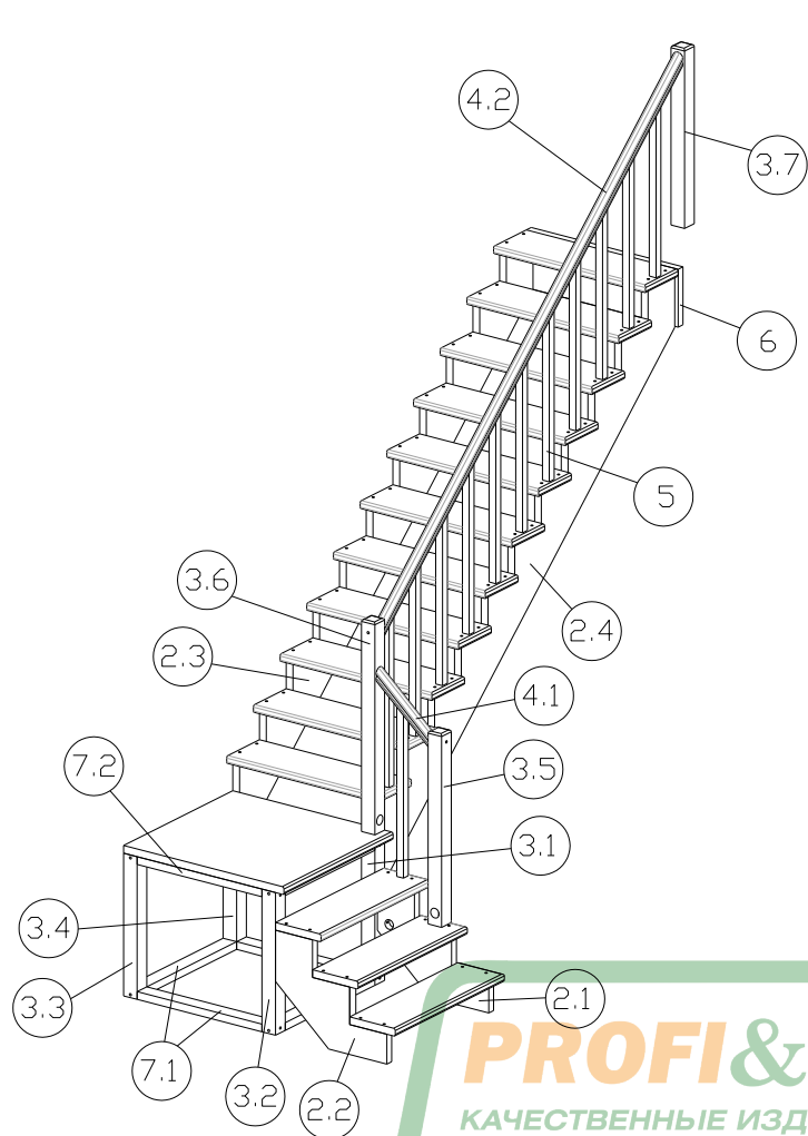
Вариант без подступеней
